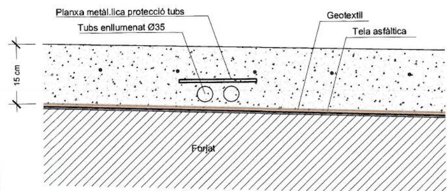
DETALL PROTECCIÓ TUBS ENLLUMENAT A1 e:1/5 A3 e:1/10
