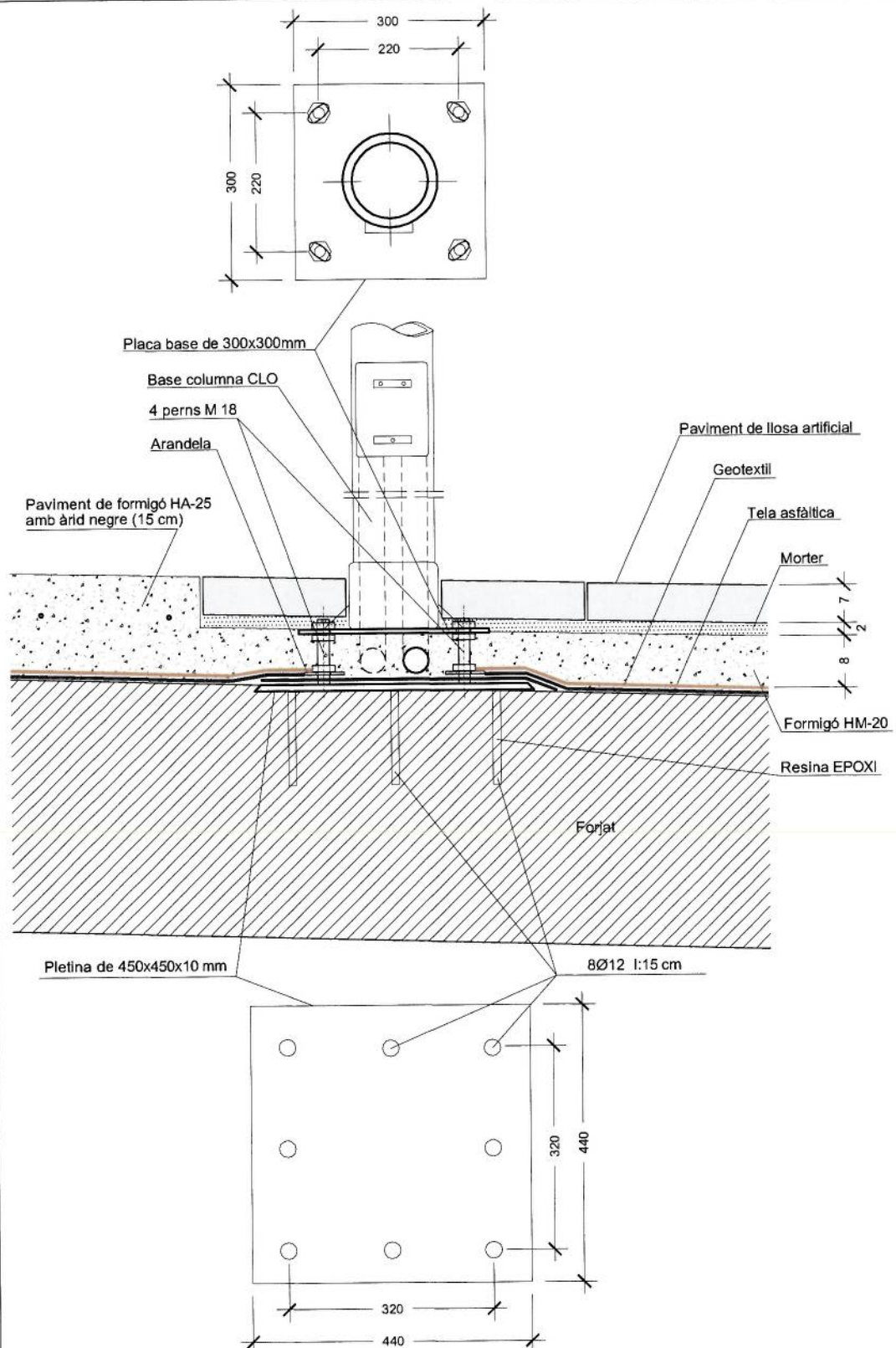
DETALL BASE FAROLA SOBRE PAVIMENT A1 e:1/5 A3 e:1/10
