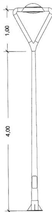
DETALLS LLUMINARIA HEKA LH D'IEP (SIMON LIGHTING) Vmh 70W columna especial Simon Lighting per l'Ajuntament d'Olot
