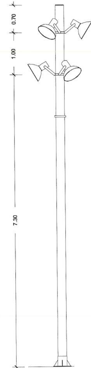
DETALLS PROJECTORS TIPUS PR31 D'IEP (SIMON LIGHTING) Vmh 150W sobre columna CL5 (Sistema Tower)
