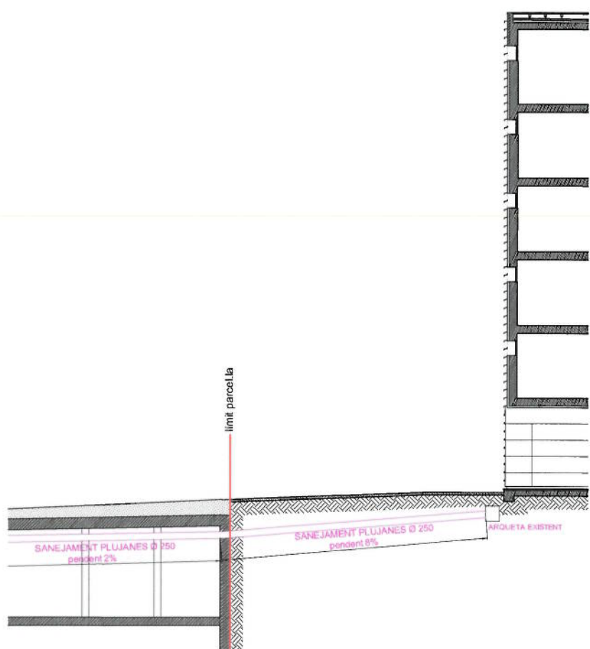
PERFIL LONGITUDINAL SANEJAMENT PLUJANES A3 e:1/100 A3 e:1/200
