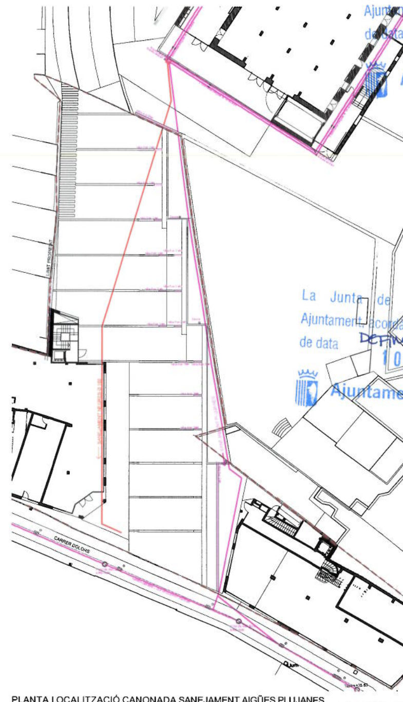
PLANTA LOCALITZACIÓ CANONADA SANEJAMENT AIGÜES PLUJANES
