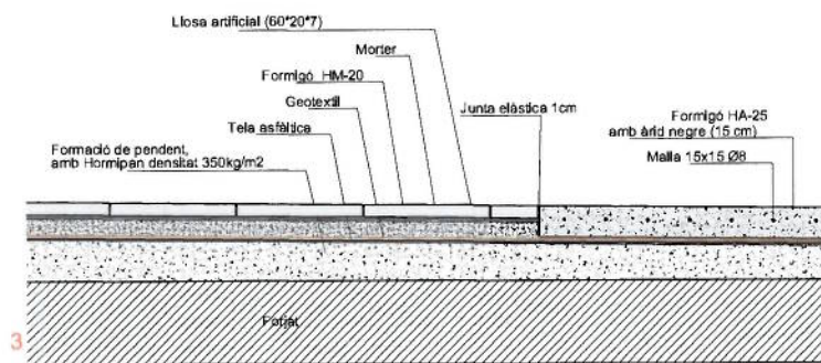
DETALLS SECCIÓ A1 e:1/20 A3 e:1/40
