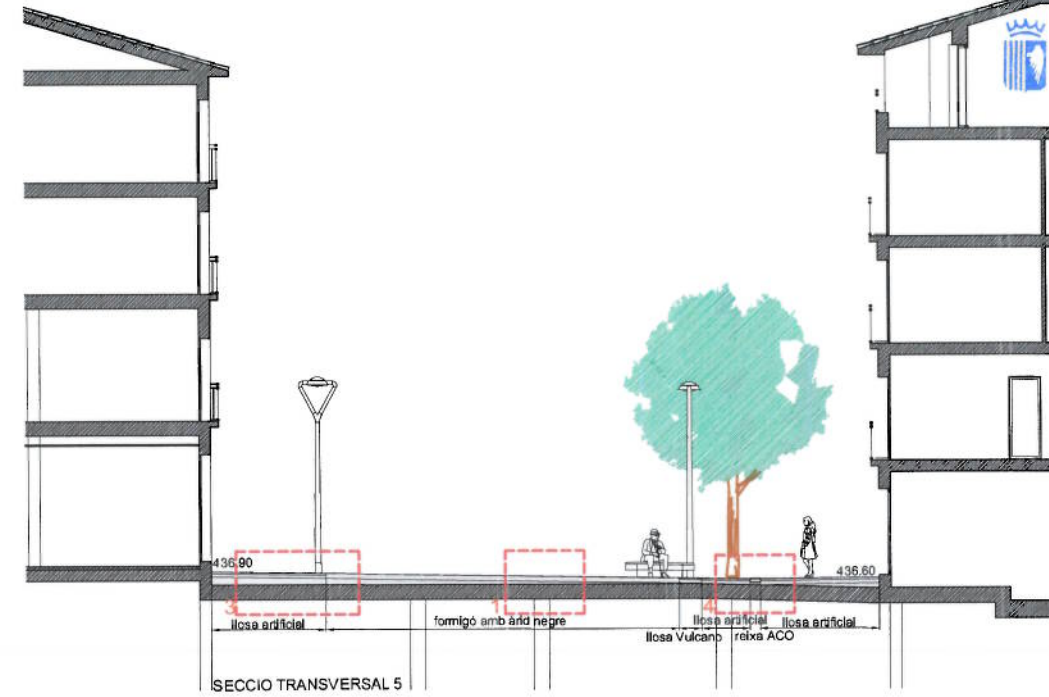
SECCIO TRANSVERSAL 5
