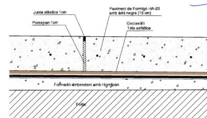
DETALLS JUNTA DE DIL-LATACIÓ TIPUS (C) JUNTES PAVIMENT A1 e:1/5 A3 e:1/10
