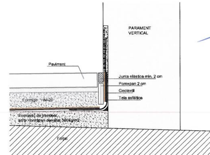
DETALL JUNTA DIL-LATACIÓ TIPUS (B) TROBADA PAVIMENT AMB PARAMENT VERTICAL A1 e:1/5 A3 e:1/10
