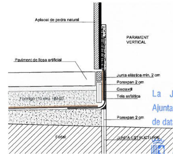
DETALL JUNTA DIL-LATACIÓ TIPUS (A) PAVIMENT A JUNTA ESTRUCTURAL A1 e:1/5 A3 e:1/10
